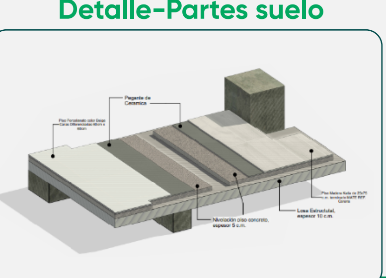
Detalle-Partes suelo
