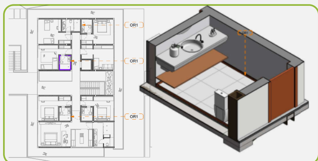
Detalles perfiles
