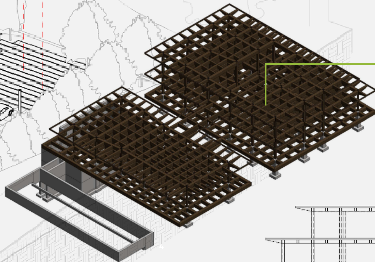
Modelo Estructural
